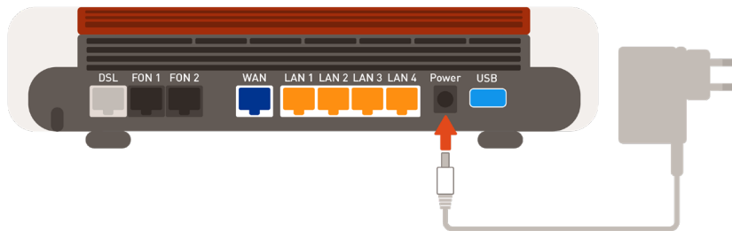
Anschließen der Stromversorgung
